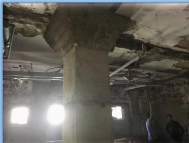
مقاوم سازی ستون بعد از اجرا
